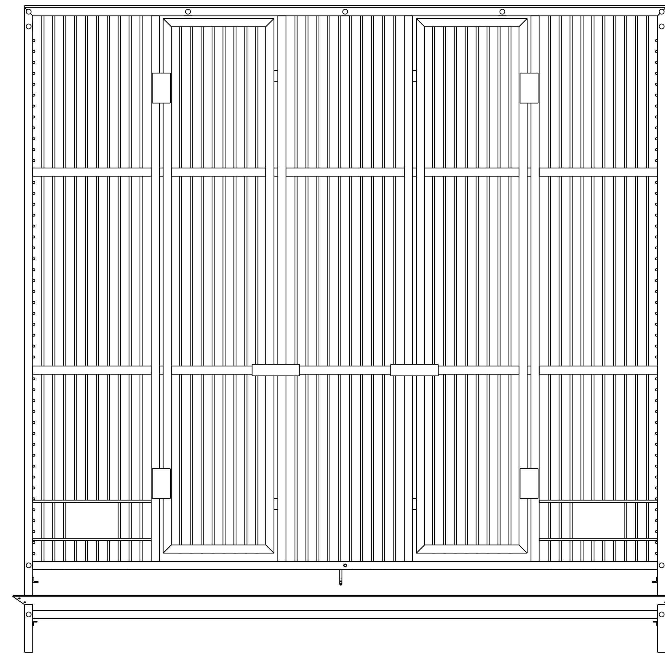
Přední pohled (skryty zadní dráty pro lepší orientaci)
