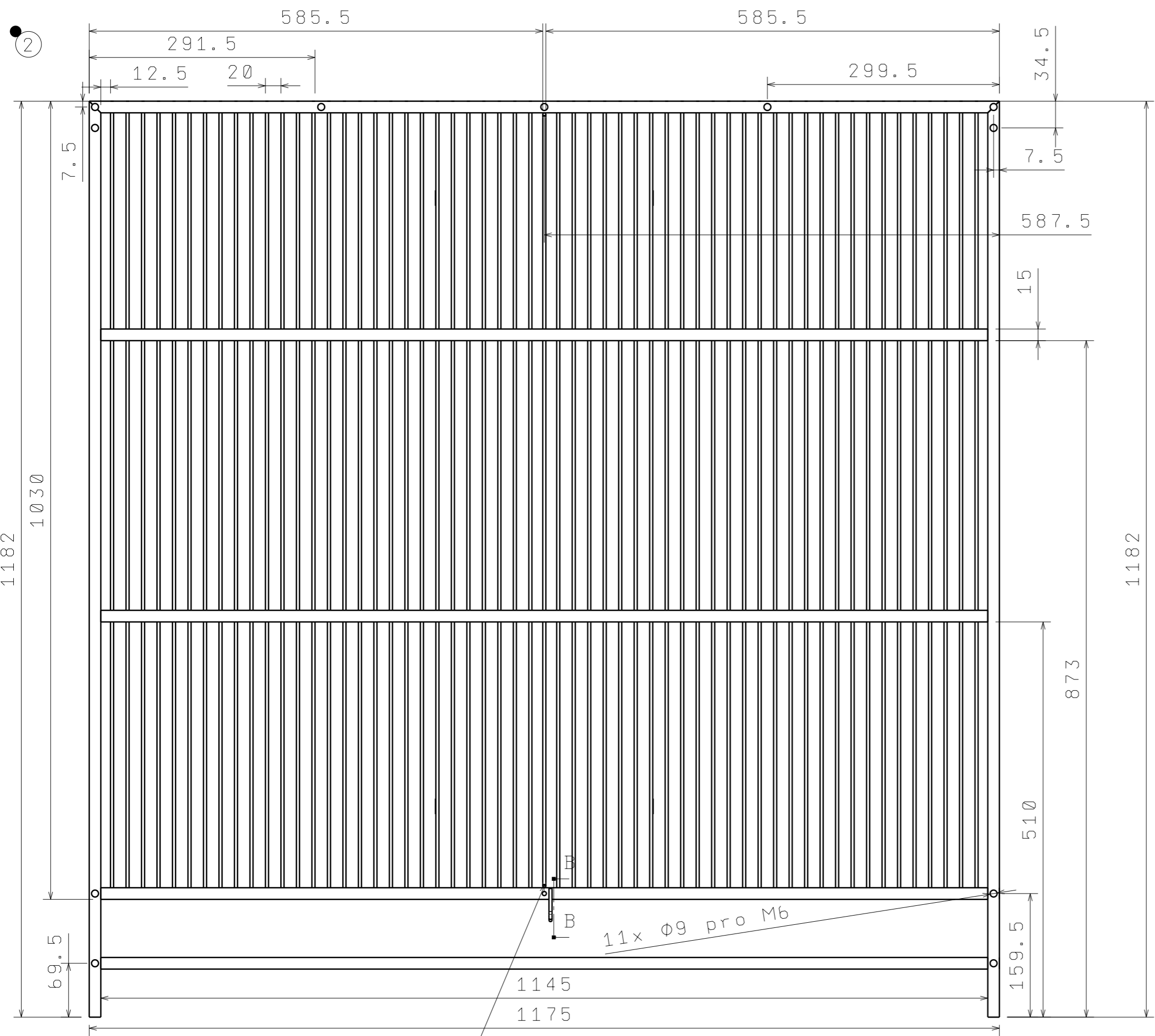
Zadní panel (pohled ze zadu z venku) 1:5
